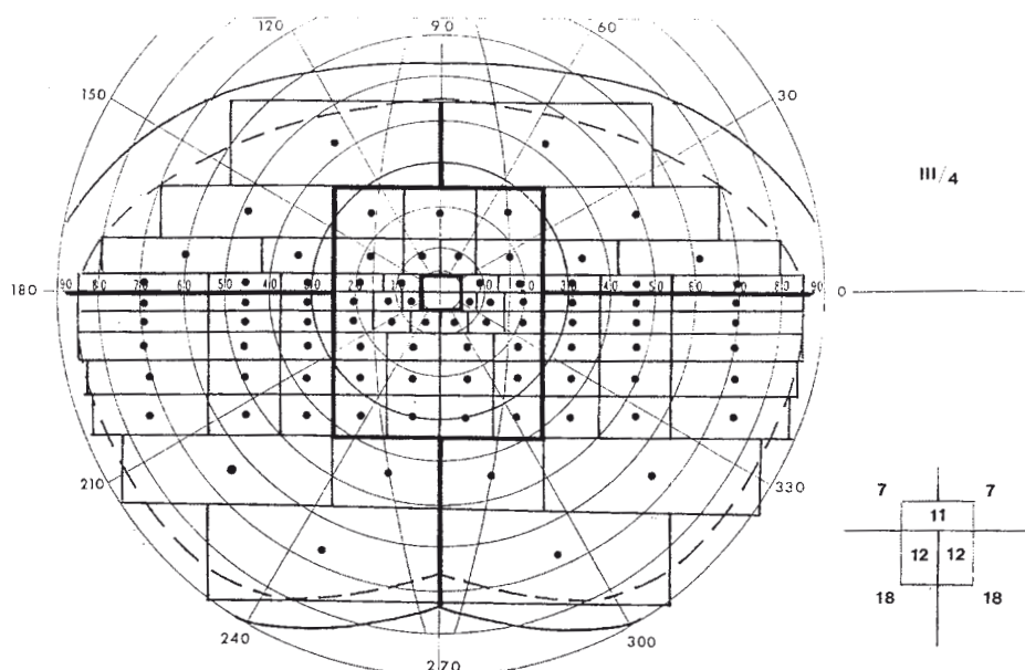
Schéma 1 Approche de l'indemnisation du champ visuel (la ligne brisée représente la limite du champ visuel binoculaire normal pour l'isoptère III/4). Chaque point correspond à une lacune non perçue et à 1% d'IPP.
